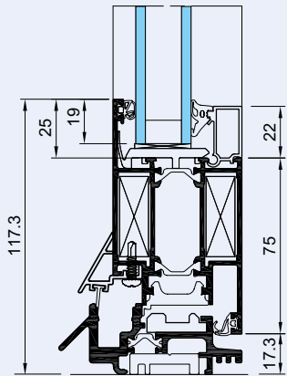
Seuil PMR démontable de 20 mm "résidentiel", ouverture intérieure uniquement
