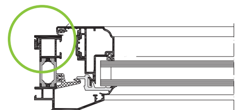
Coupe technique de la bicoloration rapportée
