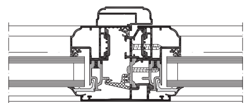
Poignée centrée
